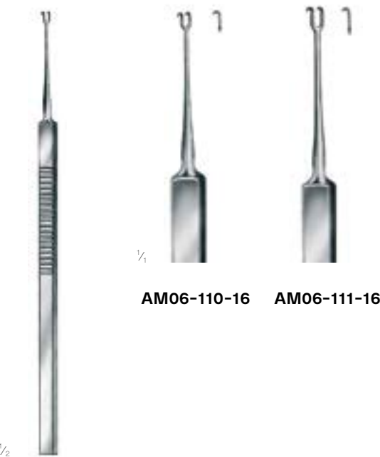
Guthrie AM06-110-16 AM06-111-16 15,5 cm / 6 1/8" sharp
